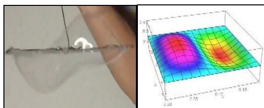
圖 8：振動鐵絲框的方形肥皂膜駐波及模擬圖形
