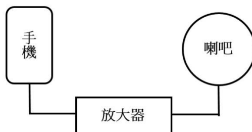
圖 1：肥皂膜實驗接線圖
