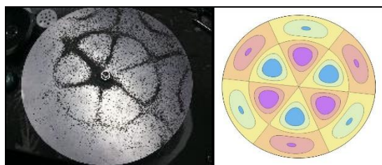
圖 11：圓形金屬片振動的高階駐波及其模擬圖
