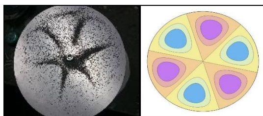
圖 10：圓形金屬片振動的低階駐波及其模擬圖
