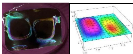
圖 4：頻率為 23 Hz 的方形肥皂膜駐波及模擬圖形
