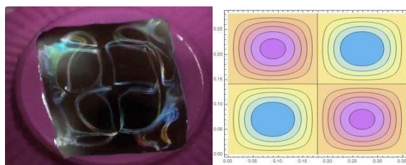
圖 5：頻率為 46 Hz 的方形肥皂膜駐波及模擬圖形
