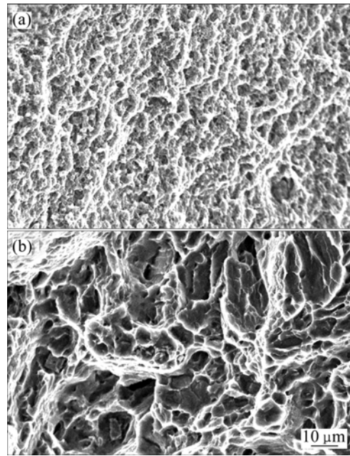
图8 Mg-Ti复合层拉伸断口的SEM像
