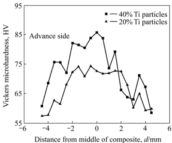
图 5 Mg-AZ31/Ti 复合层区显微硬度分布曲线
