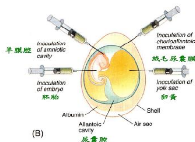
圖 3-10 以雞胚胎培養動物病毒。(A) 不同病毒打入雞胚之不同部位如圖(B)所示，病毒可在其內繁殖。
